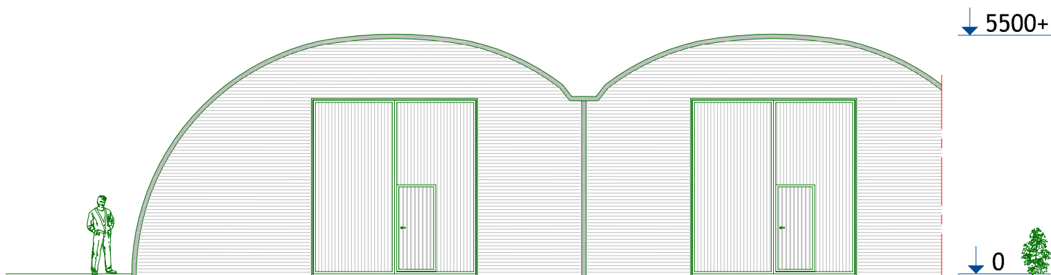
Sliding door 3750x4000 Sliding on inside Sliding door 3750x4000 Sliding on inside Schiebetor, Innenlaufend / Schuifdeur, binnenschuivend Schiebetor, Innenlaufend / Schuifdeur, binnenschuivend
