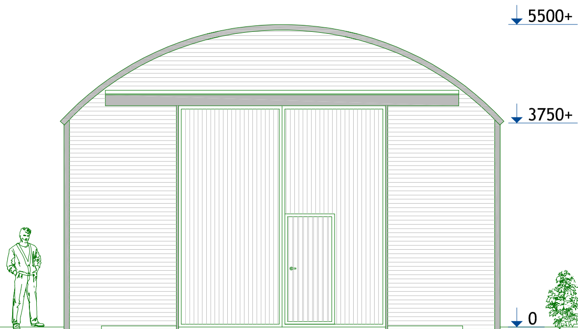
Sliding door 3750x4000 Sliding on outside Schiebetor, Außenlaufend / Schuifdeur, buitenscheuwend ± 7900
